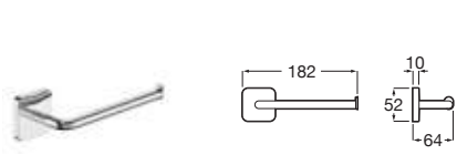
Portarrollo sin tapa
