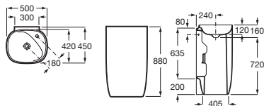
Lavabo Totem Fineceramic® Incluye desagüe universal con tapón cerámico Ø72 mm Blanco Blanco mate 500 x 450 x 880 A3270B0..0 € 1.981,00 € 2.373,00
