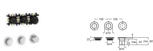
Grifería termostática empotrable 2 vías A completar con cuerpo empotrable
